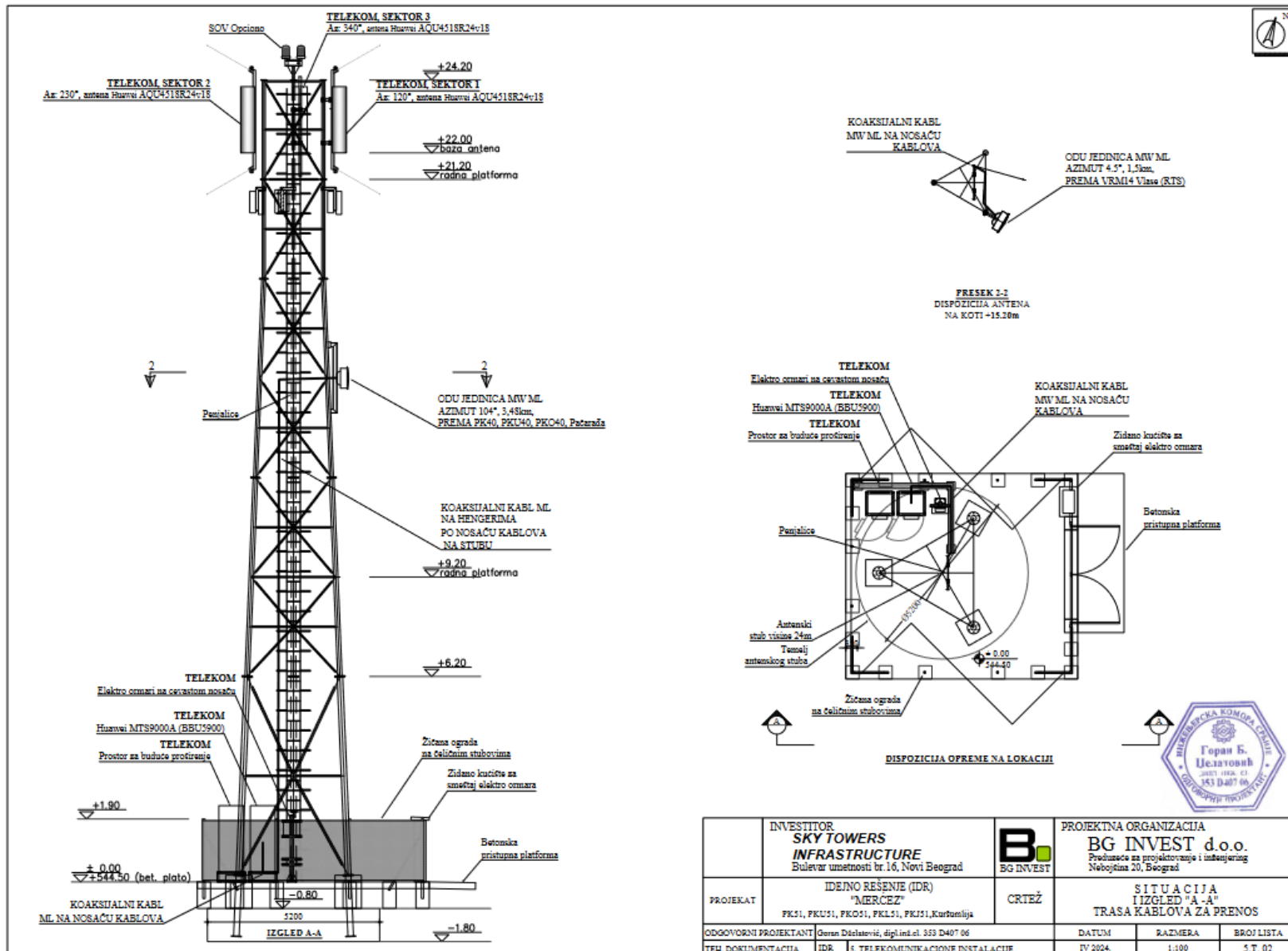
Слика 3.2. Идејно решење – ситуација и изглед „А-А“ – траса каблова за пренос
