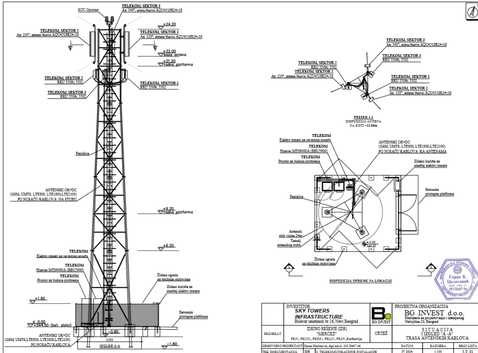
Слика 3.1. Идејно решење – ситуација и изглед „А-А“ – траса антениских каблова
