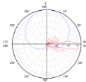
690-960 MHz (Lr1/Rr2)
